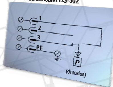
2. Anschlussbild DS-502
